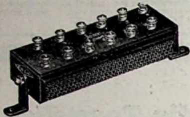
BULGIN 20.000 Ohms P.O. Meter vullige doorlaat 40 Milliamps. f 4.50 per stuk met schema
